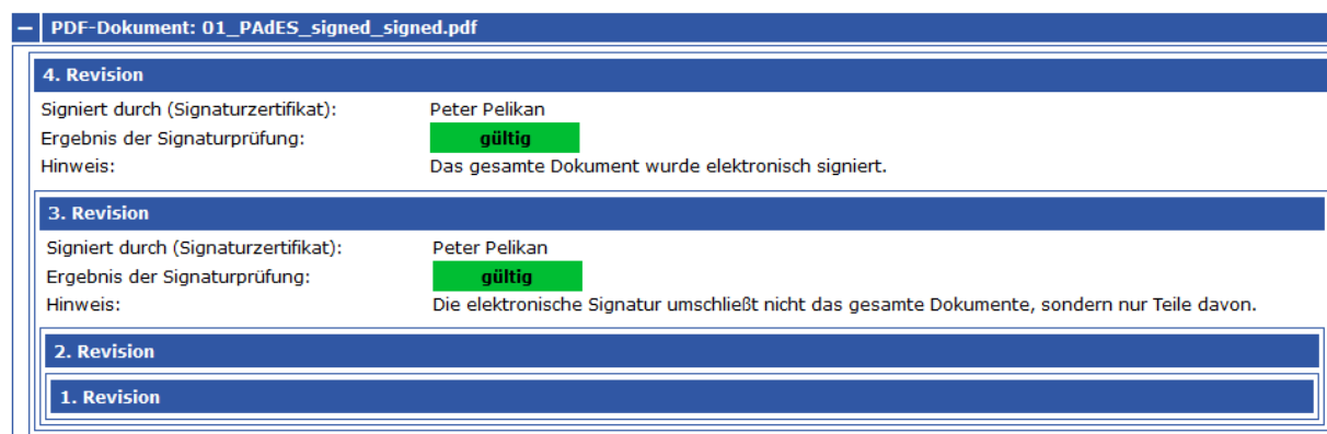
Abbildung 29: Bereich A "Dokument-/Containerstruktur" (aufgeklappt) bei einem signierten PDF-Dokument mit zwei Signaturen
