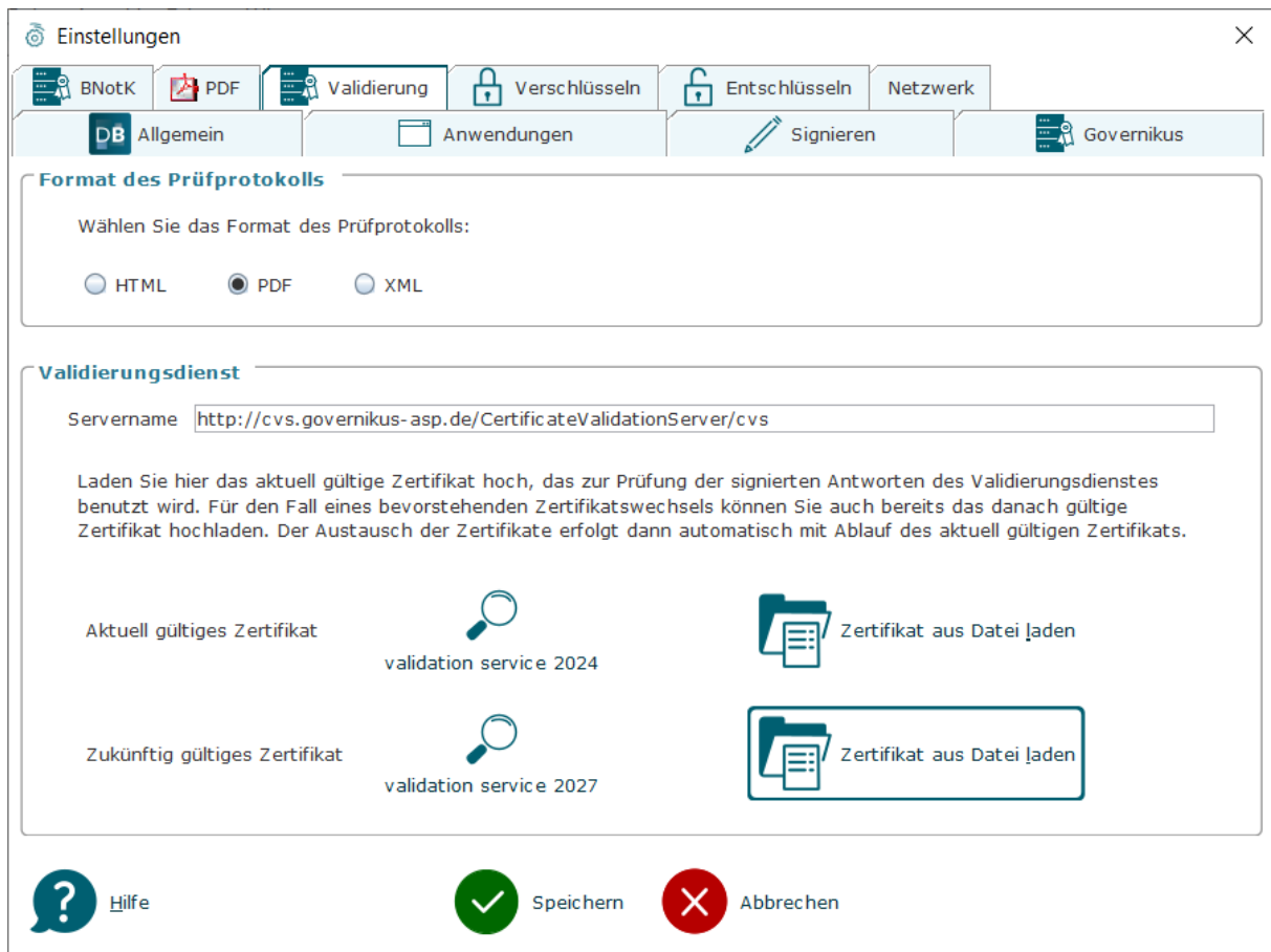
Abbildung 26: Registerkarte Validierung
