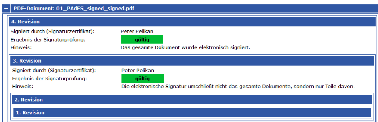
Abbildung 19: Bereich A "Dokument-/Containerstruktur" (aufgeklappt) bei einem signierten PDF-Dokument mit zwei Signaturen
